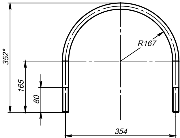
Поз.5 (Хомут)
