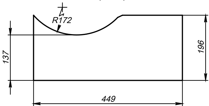
Поз.2 (Угольник) развертка
