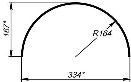
Поз.6 (Прокладка)
