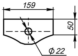
Поз.4 (Ушко) развертка
