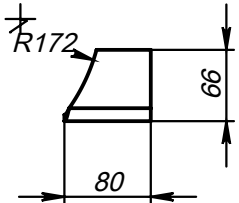
Поз.4 (Ушко)
